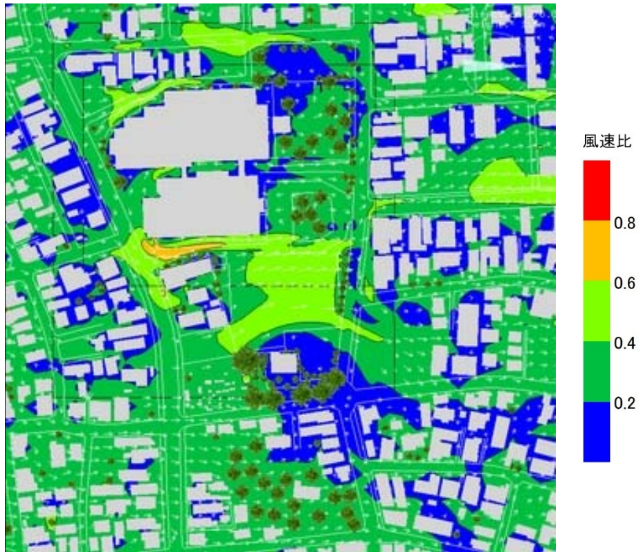
図-6 風速比 (1) 建設前、風向: 西
