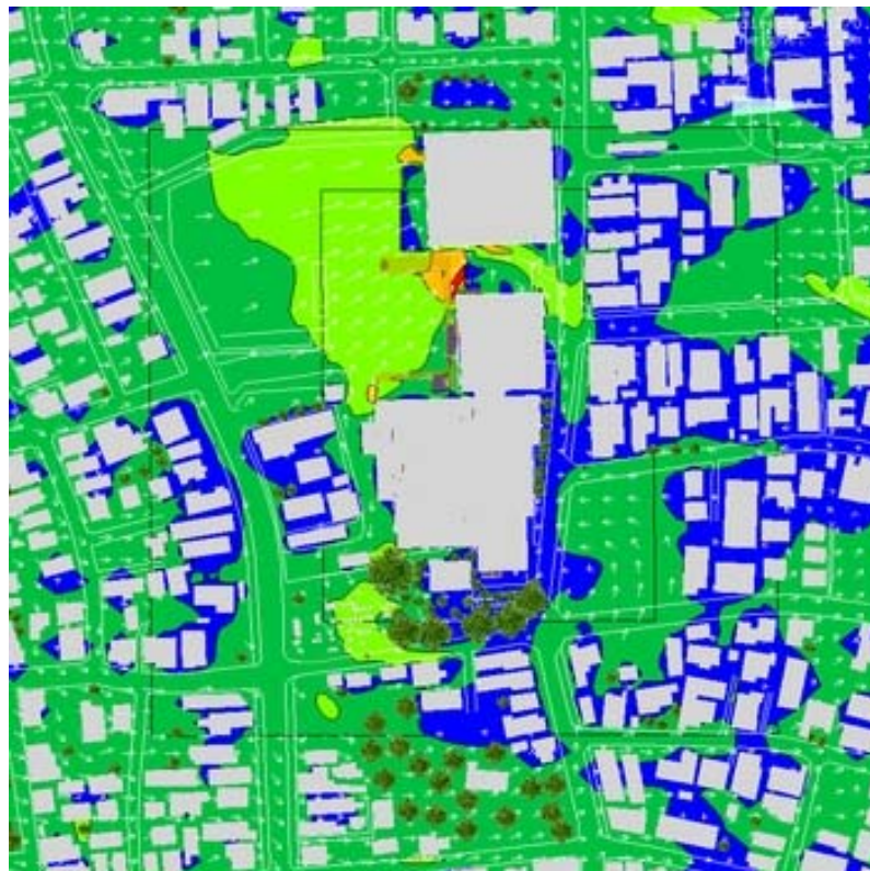
図-6 風速比 (2) 建設後、風向: 西
