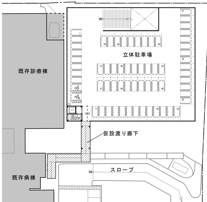
2階・屋上階平面図 S=1/800
