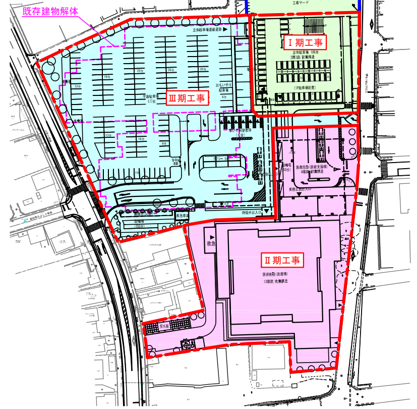
工事区分図
